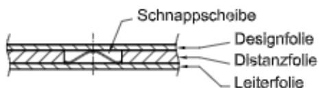
Folientastaturaufbau mit Kontaktfeder: Kontaktfeder:
